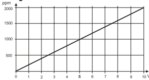
Diagramm CO 2 - Fühler
