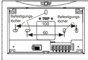
Wandschalter
